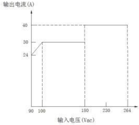
■ 降额曲线
