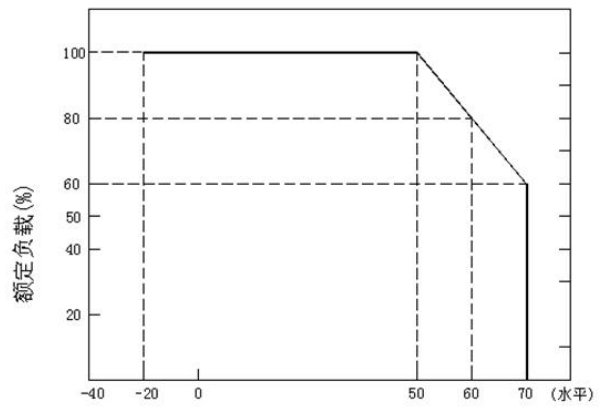
■ 环境温度VS额定功率降额曲线
