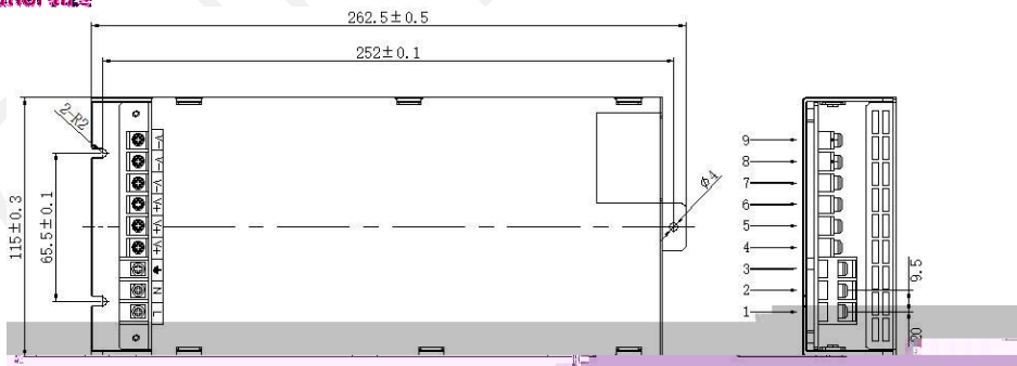
端子脚位定义
