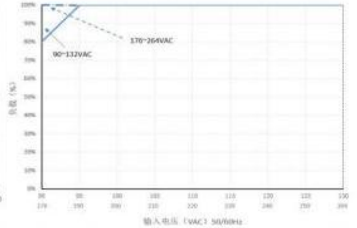
负载vs输入电压
